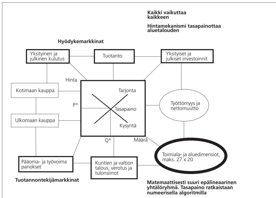
Kuva 3. RegFin-aluemallin rakenne.
